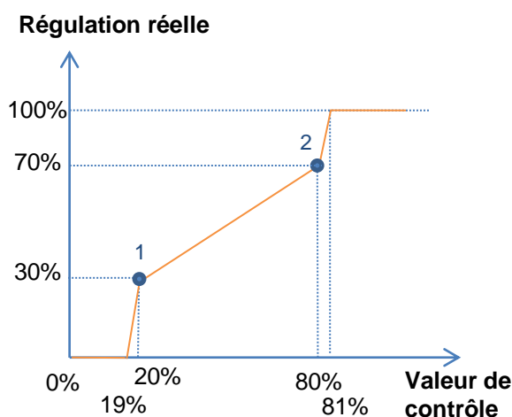
Figure 14 Courbe caractéristique - Valeurs en dehors de l'échelle.
