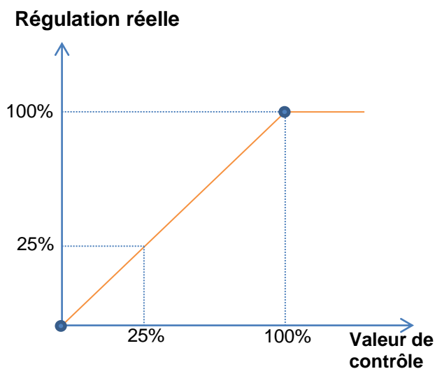
Figure 12 Courbe de contrôle par défaut.
