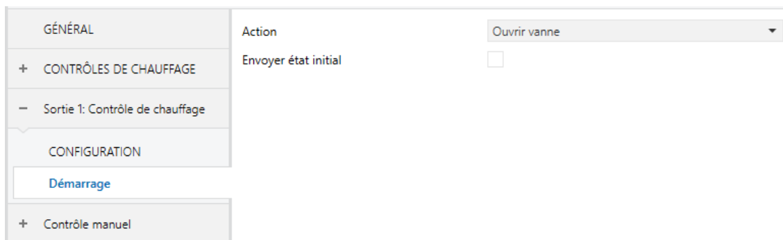
Figure 11 Contrôle de chauffage - Démarrage.
