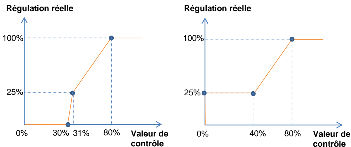
Figure 13 Courbes de contrôle personnalisées.
