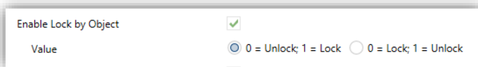
Figure 19 Bloqueo.
