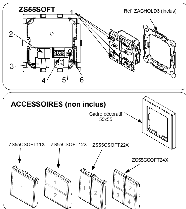
Figure 1 : Bouton poussoir Soft 55x55
