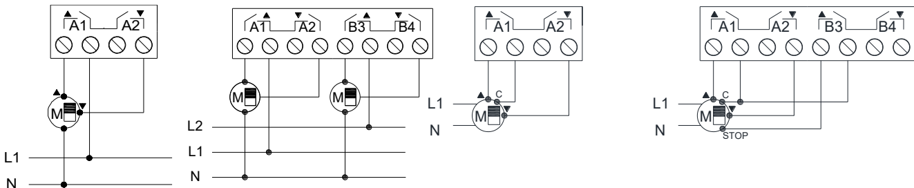
Figure 2 : Exemple de connexion (de gauche à droite) : un volet dans le canal A ; deux volets dans les canaux A et B avec des phases différentes ; un volet de 2 contacts secs dans le canal A ; et un volet de 3 contacts secs dans le canal A et sur la sortie individuelle B3
