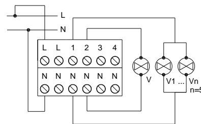
Figure 2: Exemple de connexion: une vanne par sortie et plusieurs vannes par sortie.
