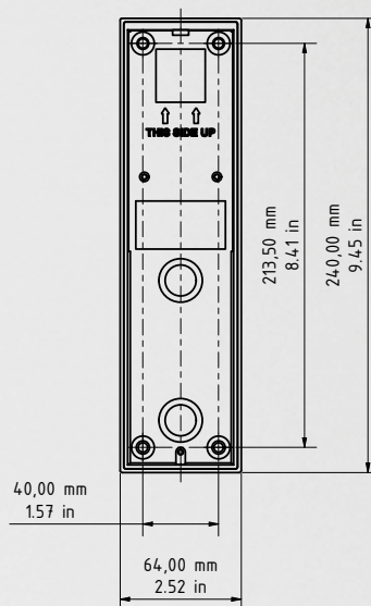
Boîtier de montage apparent
